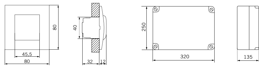
Apto para caja universal cuadrada
