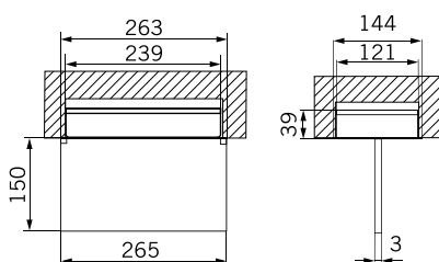
Suspendida doble / simple
