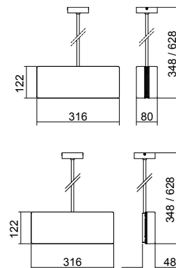
Suspendida doble / simple
