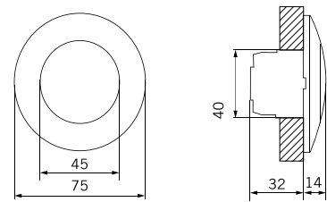
Apto para caja universal redonda
