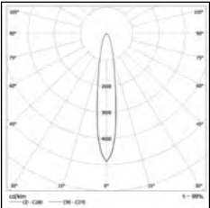
Distribución correspondiente a un solo grupo óptico orientable
