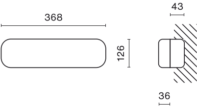
Índice: 13.5519.0002.00 Nombre: RECTANGULAR Dispositivo para empotrar. Medidas de corte según plantilla suministrada
